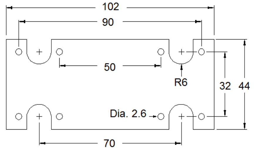
BOTTOM PCB
